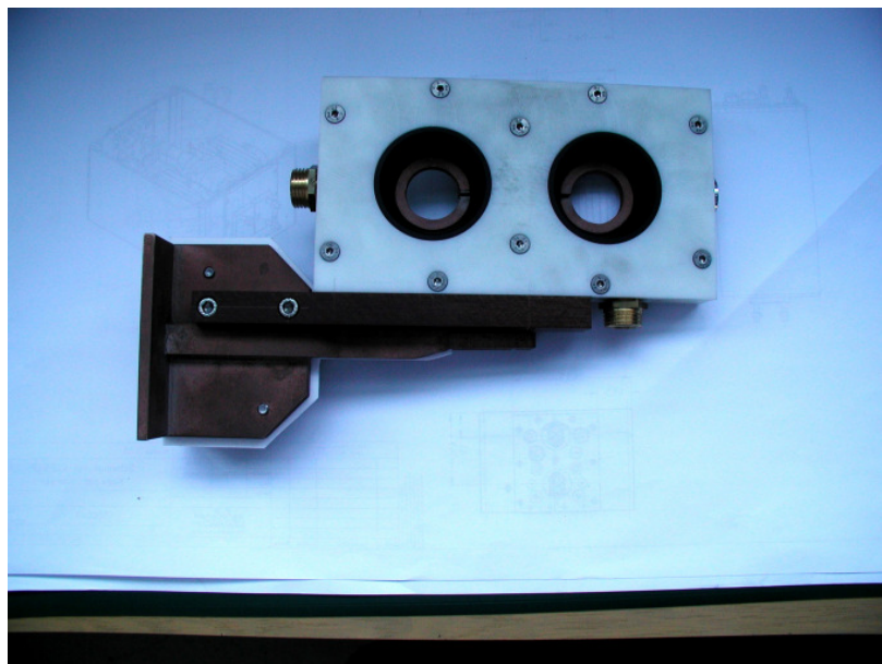
Induktor mit einer Zwillingsbrause
